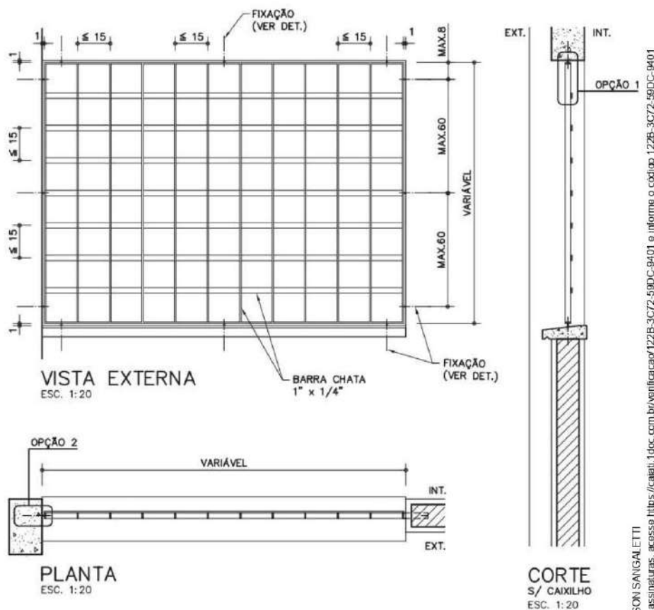
GR-01- DETALHE 02/02
