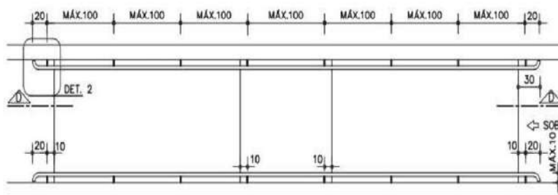
PLANTA GENÉRICA DE RAMPA
