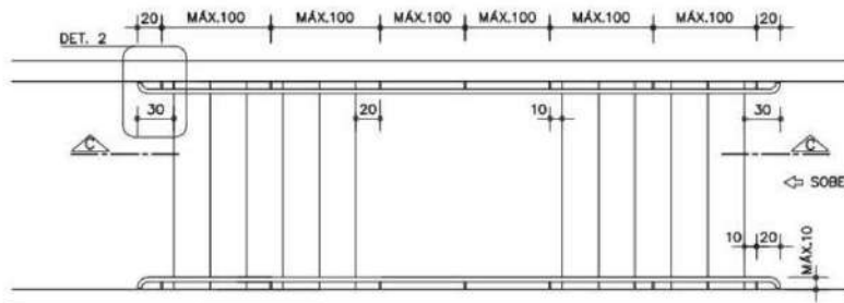
PLANTA GENÉRICA DE ESCADA
