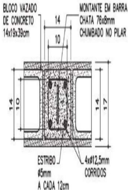
DETALHE 1 ESC. 1:10
