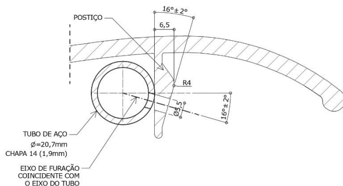
CORTE AA ESC. 1 : 1
