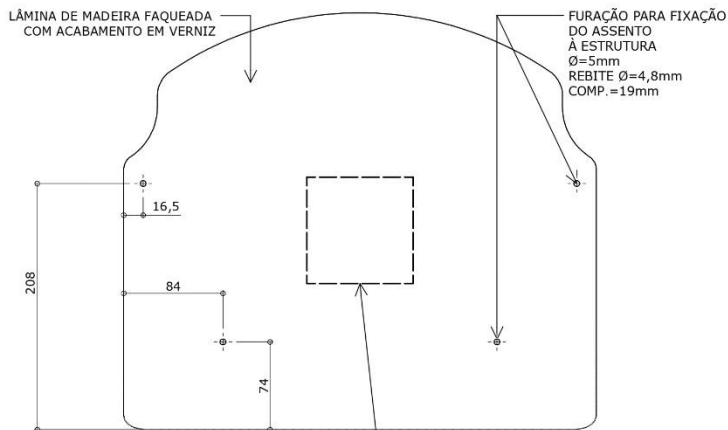
VISTA INFERIOR ESC. 1 : 5
