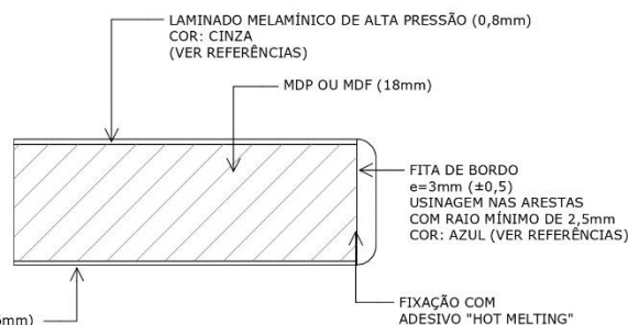
DETALHE 2 ESC. 1 : 1
