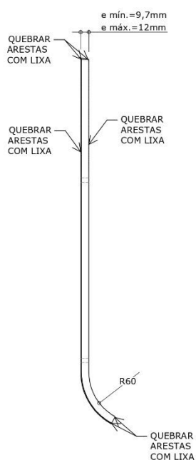
VISTA LATERAL ESC. 1 : 5
