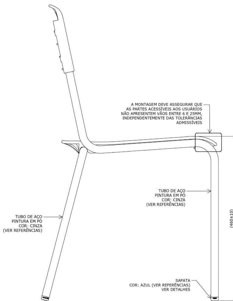
VISTA LATERAL
