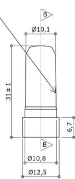
VISTA 3 ESC. 1 : 1
