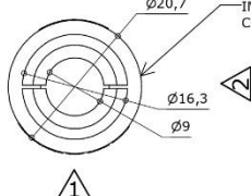
VISTA SUPERIOR ESC. 1 : 1
