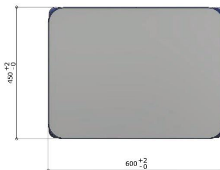
VISTA SUPERIOR ESC. 1 : 10
