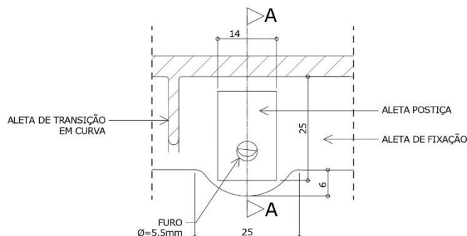
VISTA FRONTAL ESC. 1 : 1
