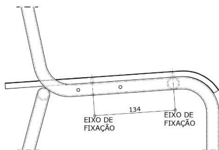
MONTAGEM ESC. 1 : 5
