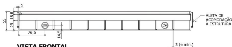
VISTA FRONTAL ESC. 1 : 5
