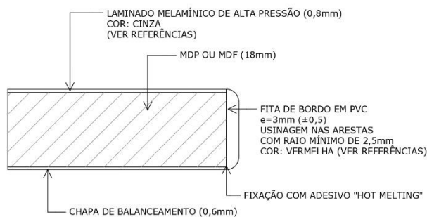
DETALHE 2 ESC. 1 : 1
