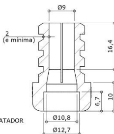
CORTE AA ESC. 1 : 1
