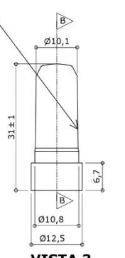
VISTA 3 ESC. 1 : 1
