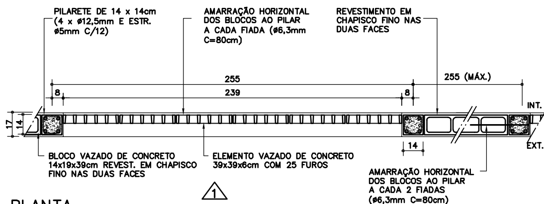
PLANTA ESC. 1:25
