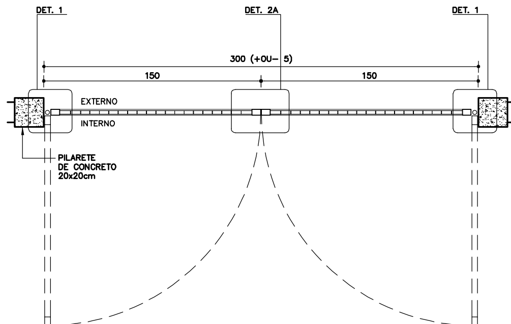
PLANTA PT-31 ESC. 1:25
