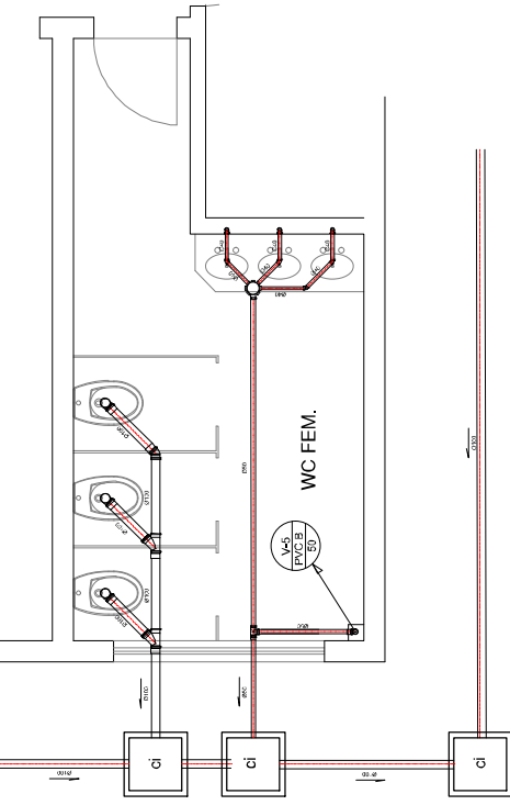
DETALHE DE ESGOTO TUBO DE 50MM Ø ESCALA 1:20
