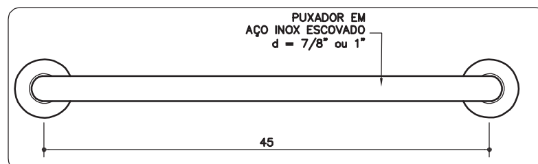
DETALHE 2 ESC. 1:5
