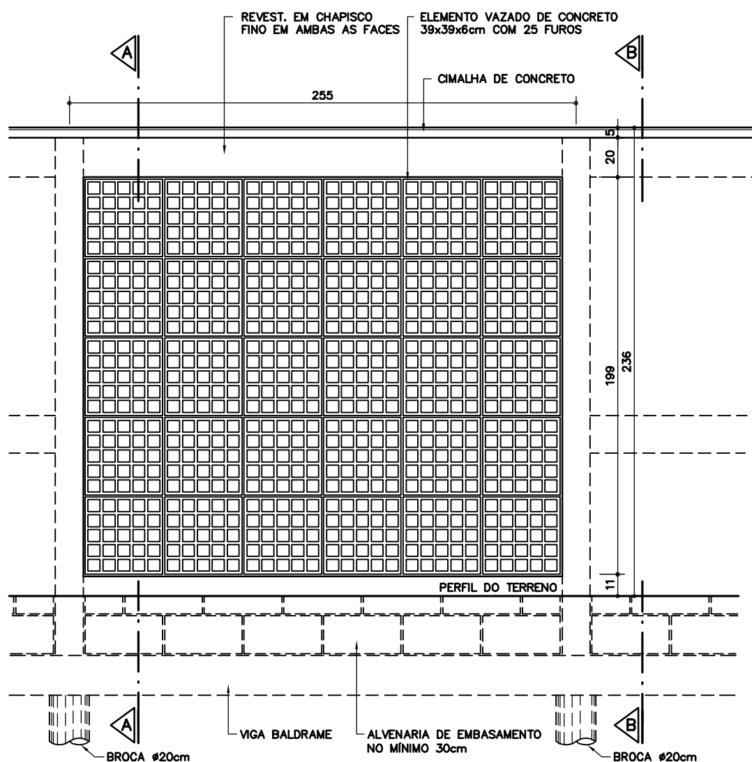
VISTA 1 ESC. 1:25
