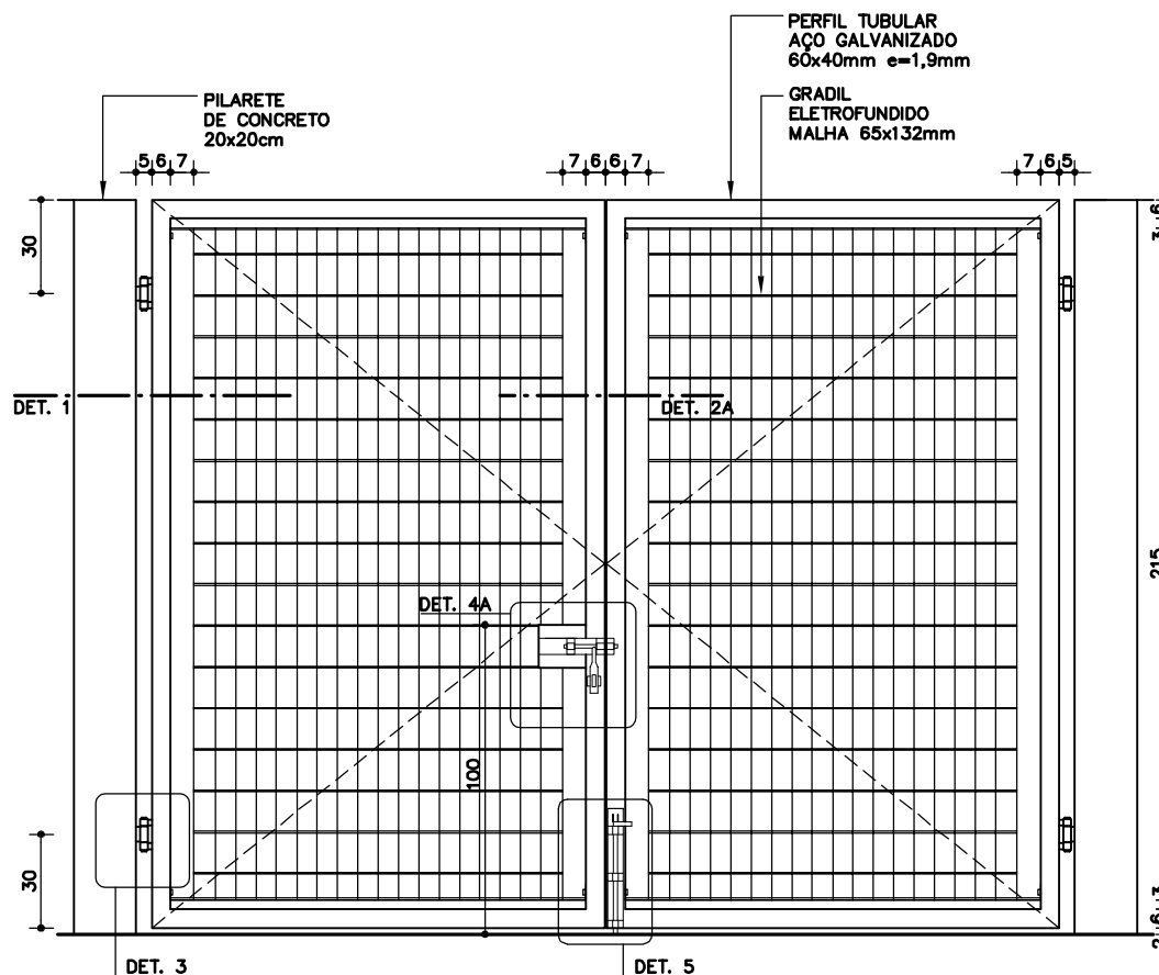
VISTA INTERNA PT-31 ESC. 1:25
