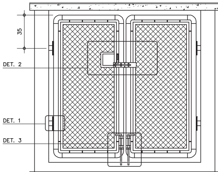
VISTA A
