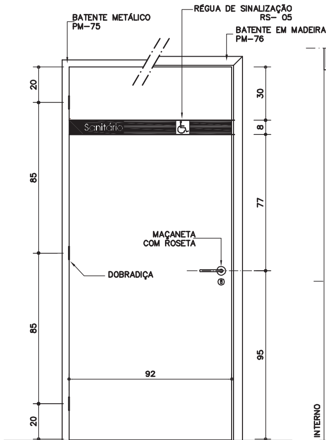
VISTA EXTERNA (1)
