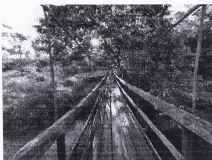
a) Visão geral da Ponte.
