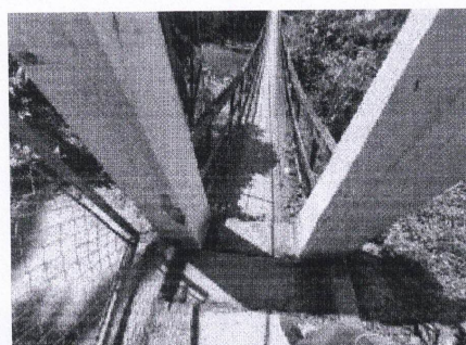
a) Pilar Danificado.
