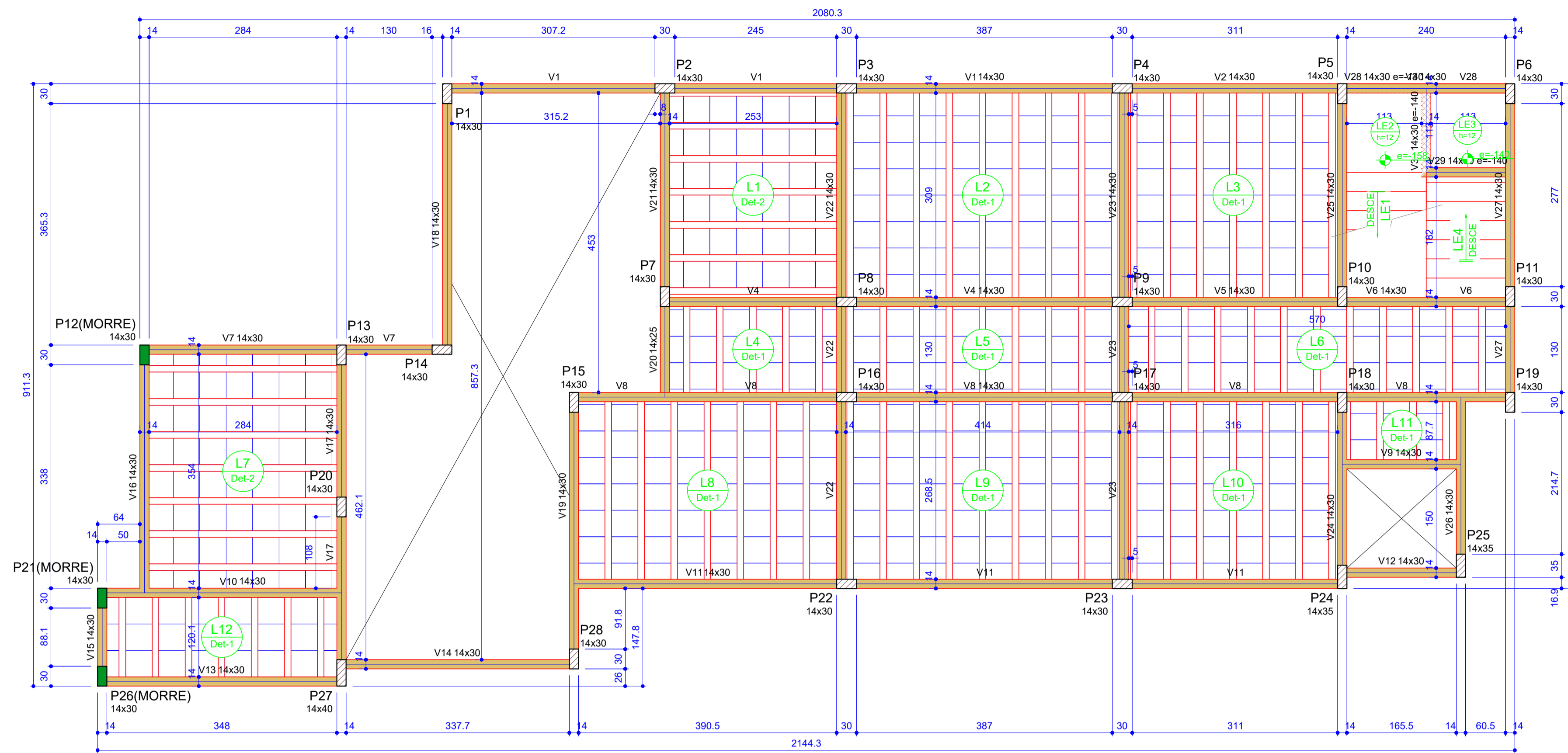
Forma do pavimento TERREO escala 1:50
