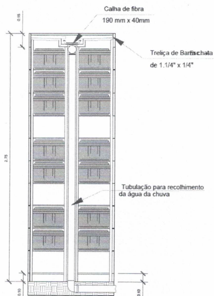
4 Corte AA Esc.: 1/10
