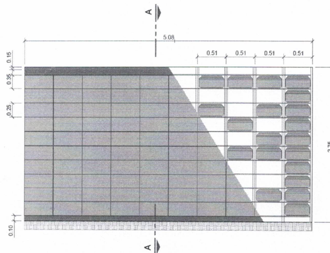
2 Vista Frontal Esc.: 1/20
