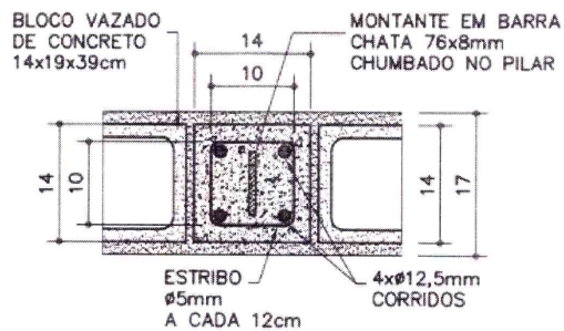
DETALHE 1 ESC. 1:10
