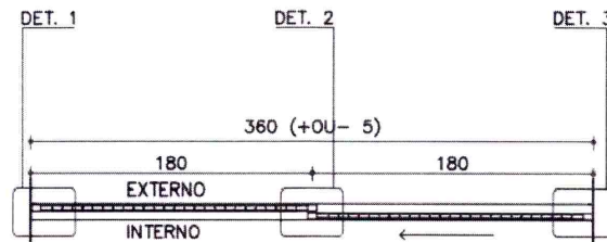
PLANTA PT-43
