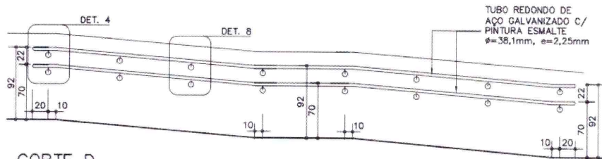
CORTE D
