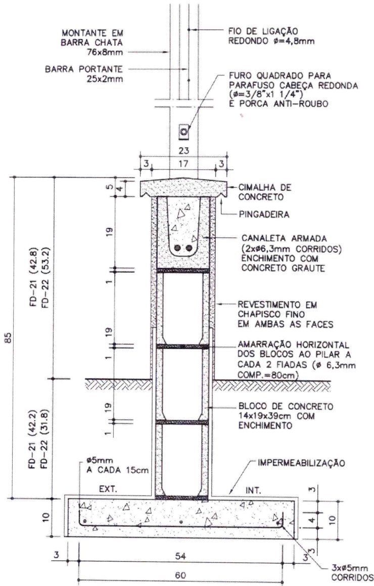
DETALHE 2 ESC. 1:10
