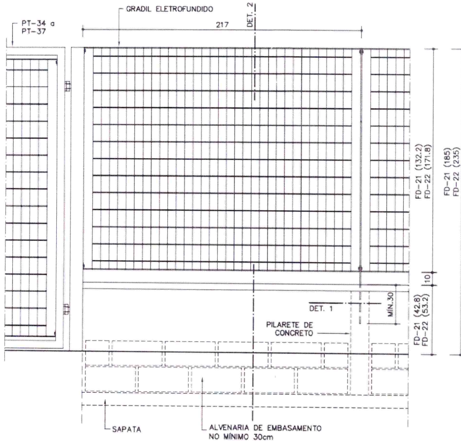
VISTA EXTERNA
