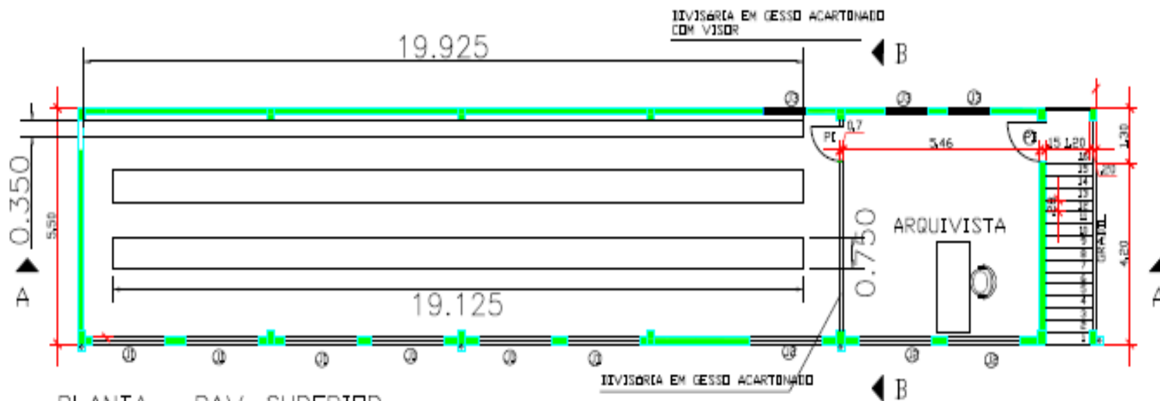
PLANTA - PAV. SUPERIOR
