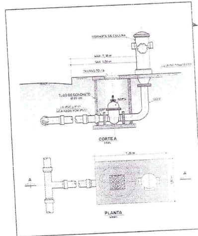
DETALHE DA INSTALAÇÃO DO HIDRANTE
