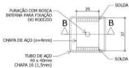
VISTA INFERIOR ESC. 1 : 2
