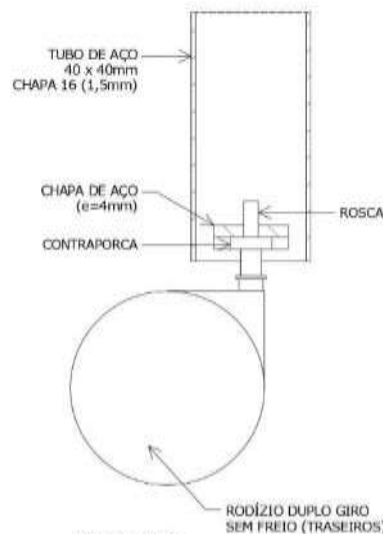
CORTE BB ESC. 1 : 2
