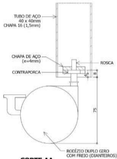
CORTE AA ESC. 1 : 2
