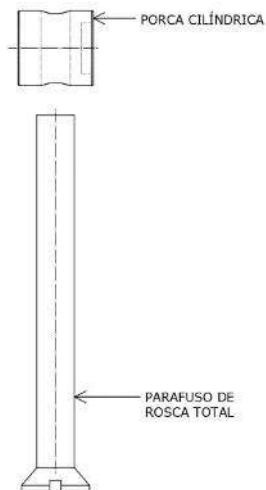
DETALHE 2 ESC. 1 : 1
